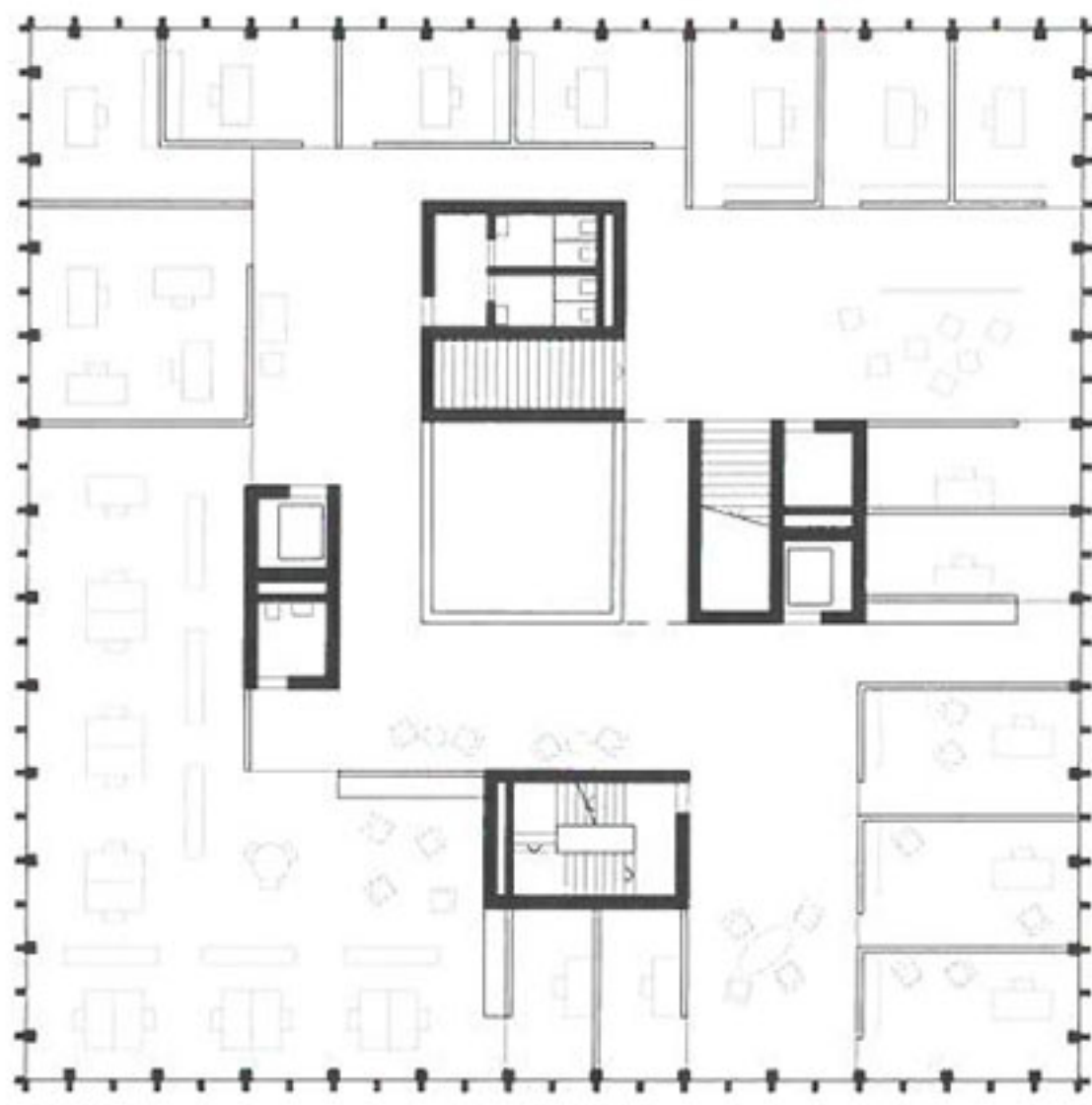
1. Obergeschoss
