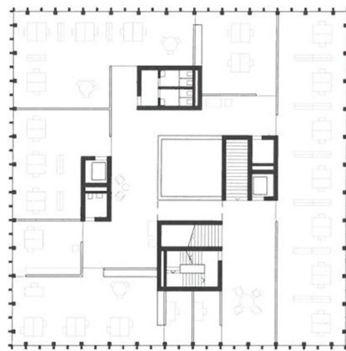
2. Obergeschoss
